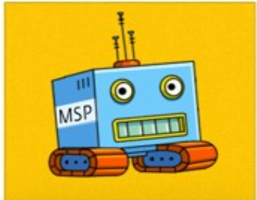
Умелый техномейкер
