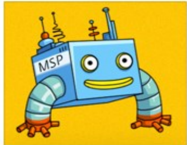
Матерый девелопер
